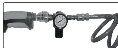
Abb. 6, Anschlusschema
